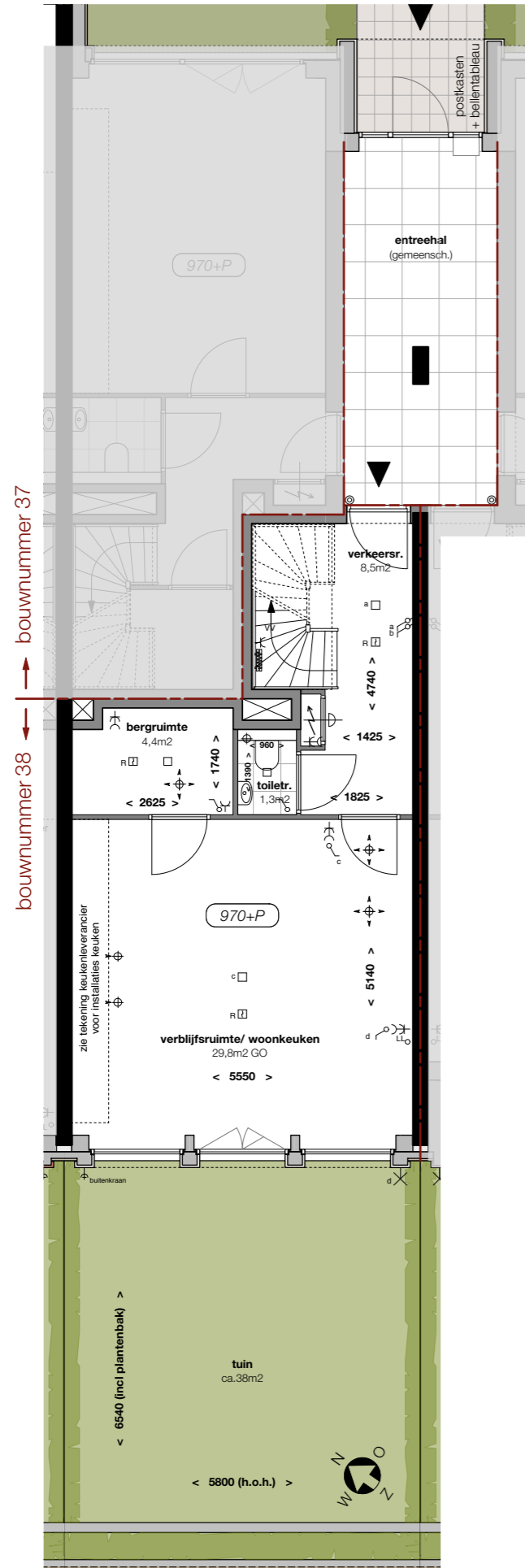
begane grond
